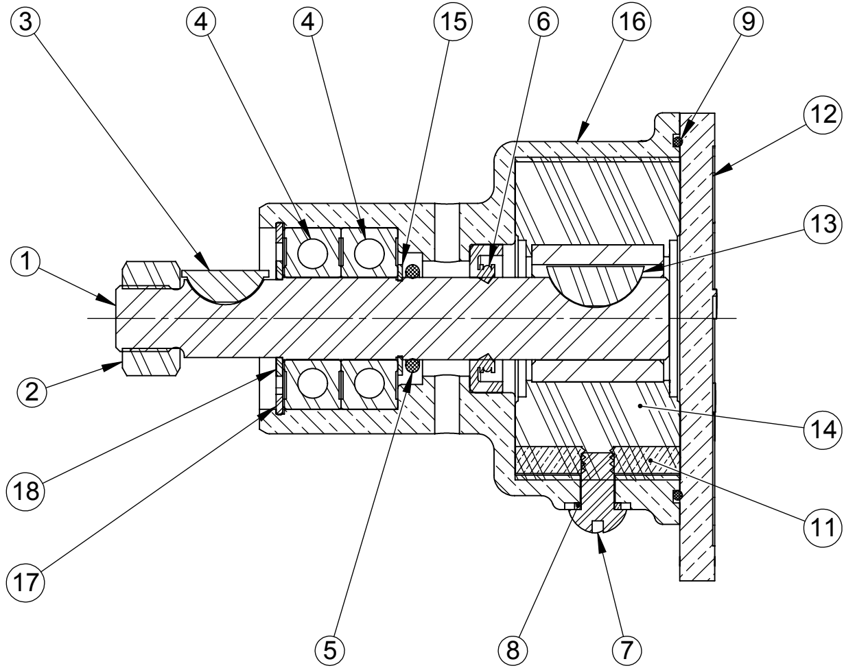
SECTION A-A
